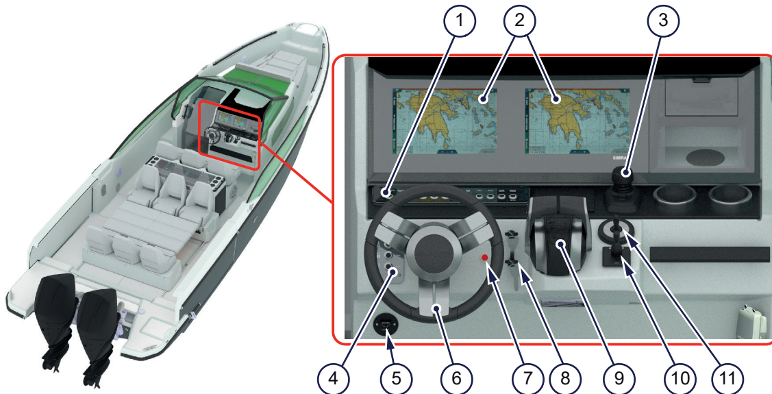
Kuva 4.3 - Ohjauspisteen hallintalaitteet
