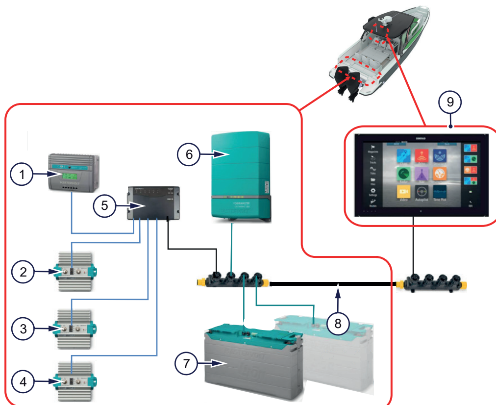
Kuva 10.4 - Tehopakettijärjestelmä
