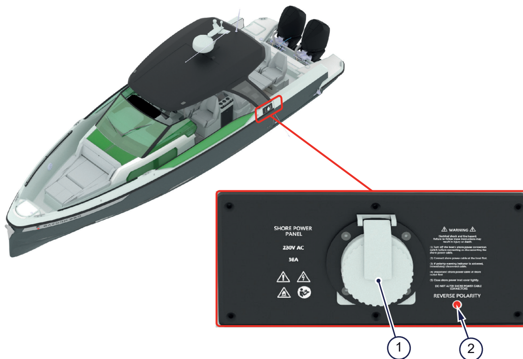
Kuva 4.10 - Maasähköpaneeli
