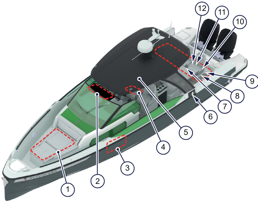
Kuva 5.1 - Sähköjärjestelmä
