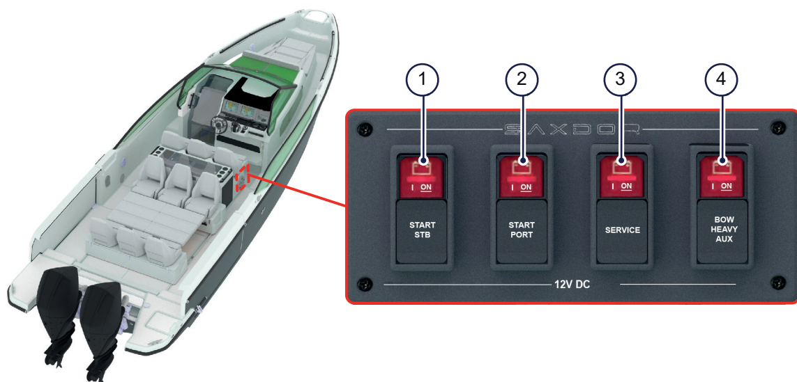
Kuva 4.9 - Akun ohjauspaneeli
