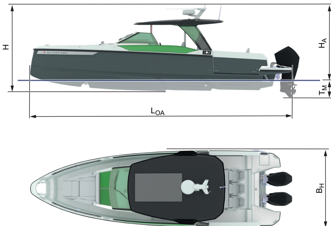
Kuva 9.1 - Saxdor 320 GTO/R:n mitat
