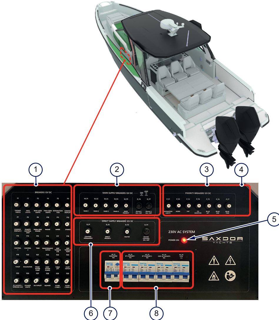
Kuva 4.8 - Etukajuutan sulaketaulu
