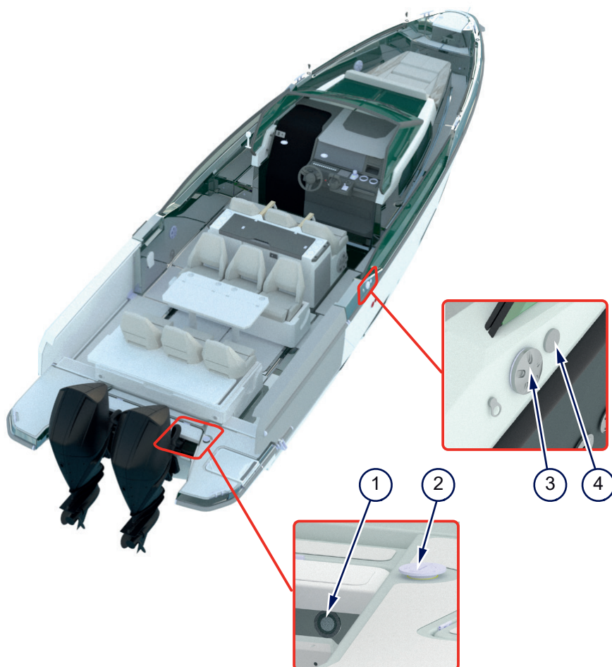
Kuva 5.3 - Polttoainejärjestelmä
